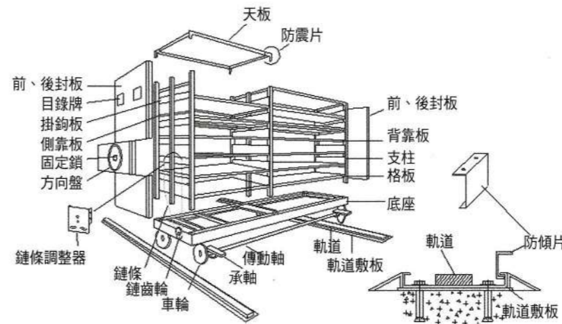
3-59 5連5層移動櫃(不含軌道) W582xD4715xH2354(mm) ◆訂購數量限1組(含)以上，15組(含)以下
