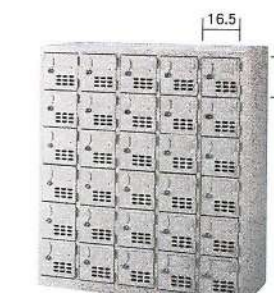
24014 30格手機櫃 W97xD35xH112.5(cm)
