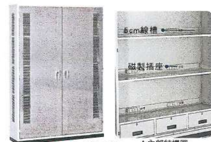
3-40 無線電櫃 W1320xD460xH1865(mm) ◆訂購數量限1組(含)以上, 50組(含)以下
