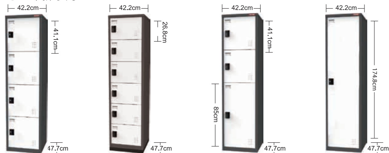
FC-104 密碼鎖 (11-13) FC-104K一般鎖 (11-17) 477W x 510D x 1800H mm
