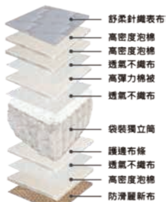
▲床墊剖面圖
