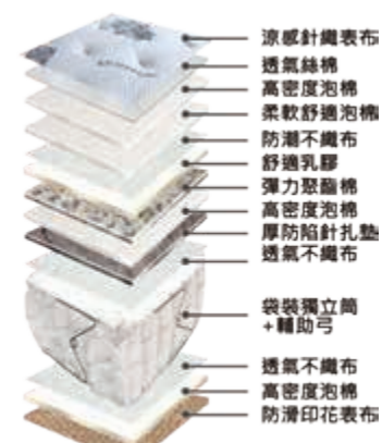
▲床墊剖面圖
