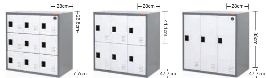
FC9-309 密碼鎖 (11-07) FC9-309K一般鎖 (11-10) 900W x 510D x 895H mm
